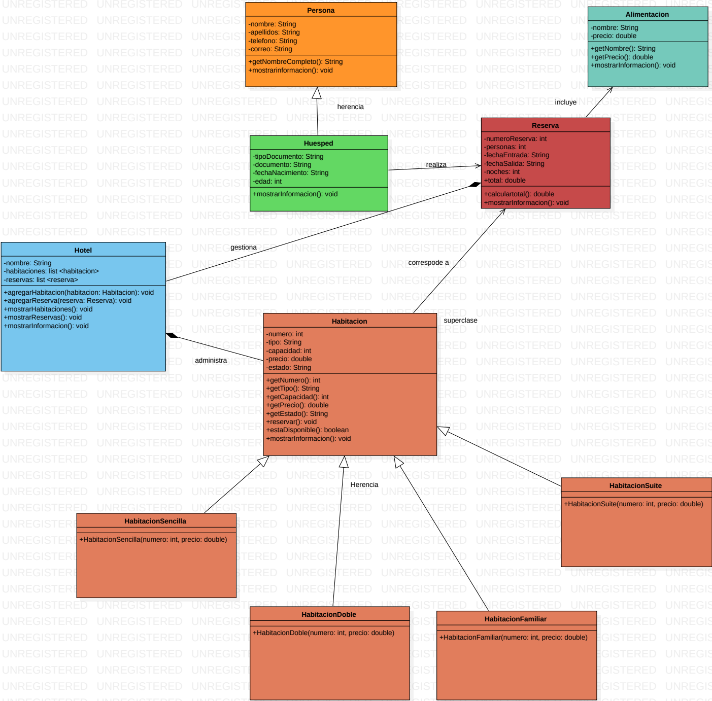
Diagrama de clases - sistema de reserva de habitaciones de hotel Paraiso
